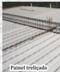
Laje treliçada
